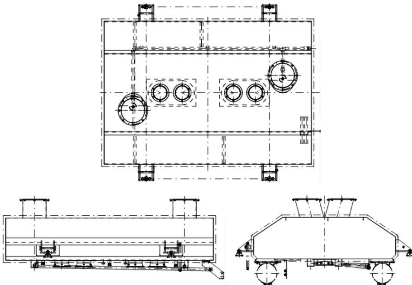
Рис. 2 – Глушитель отработавших газов дизель-локомотива проекта ВВ 475000.
