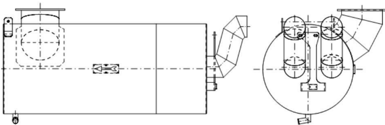
Рис. 1 – Глушитель отработавших газов дизель-локомотива проекта G-1206.
